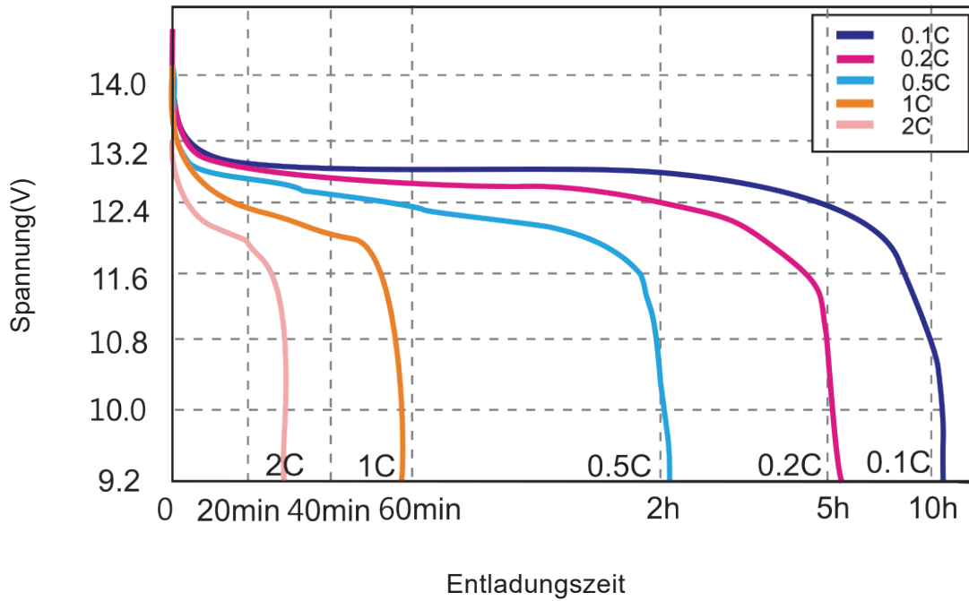
Entladekurve mit unterschiedlicher Geschwindigkeit bei @25°C
