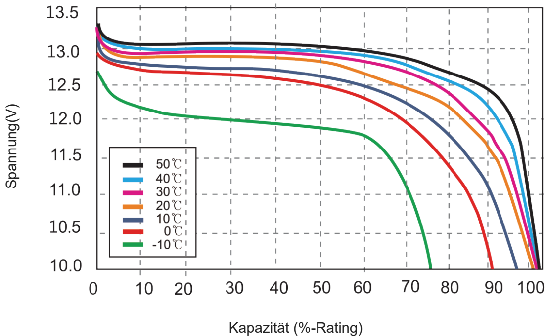
Entladekurve bei unterschiedlichen Temperaturen @0.5C
